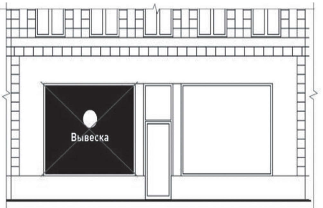
25. Размещение консольных вывесок на расстоянии менее 10 м друг от друга.
