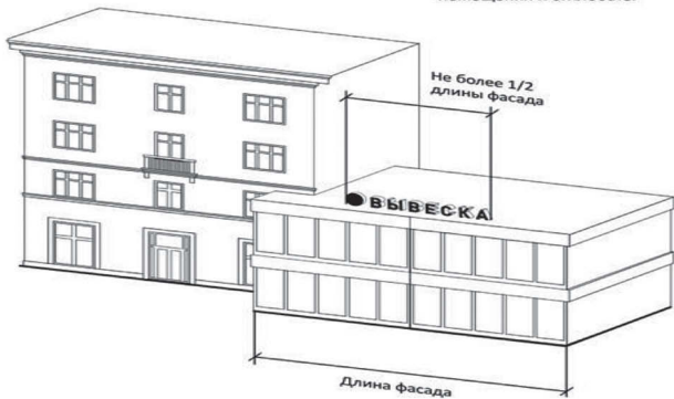
15. Нарушение геометрических параметров вывесок (пункт 48.8 Правил).
